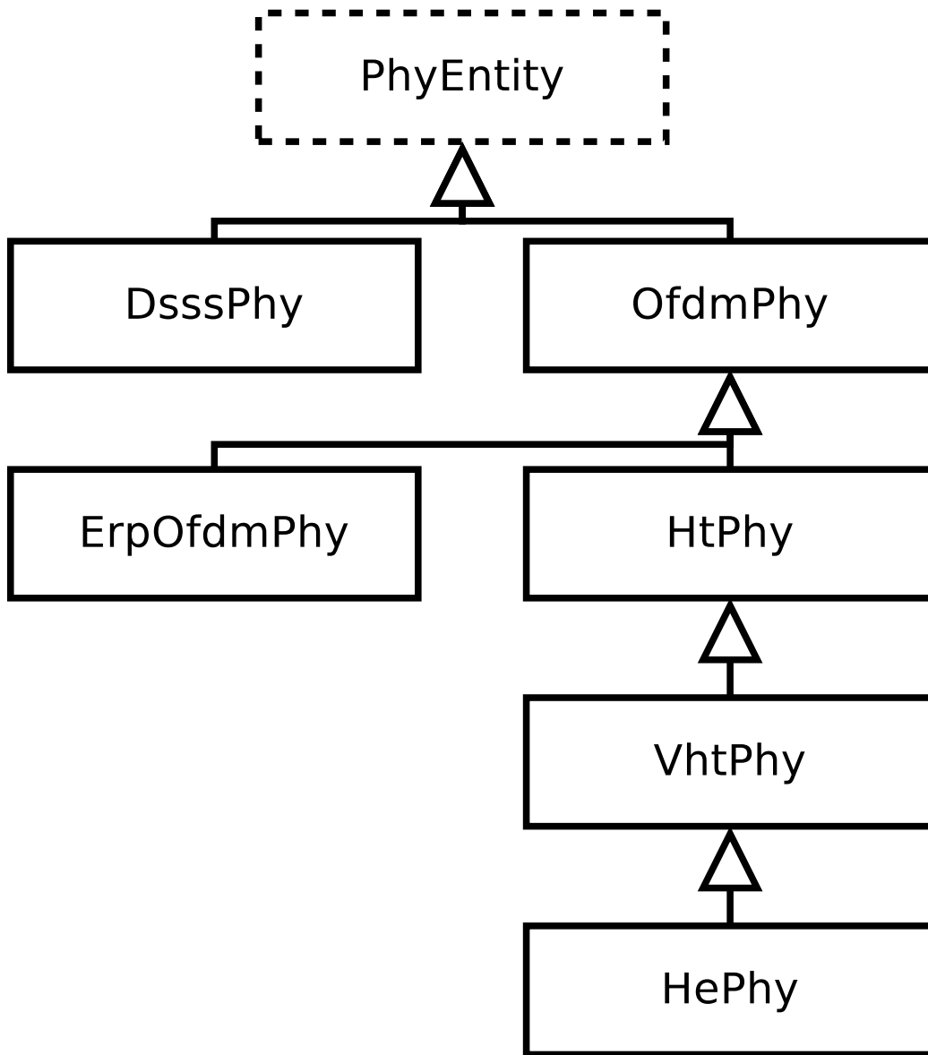
Fig. 2: PhyEntity hierarchy
