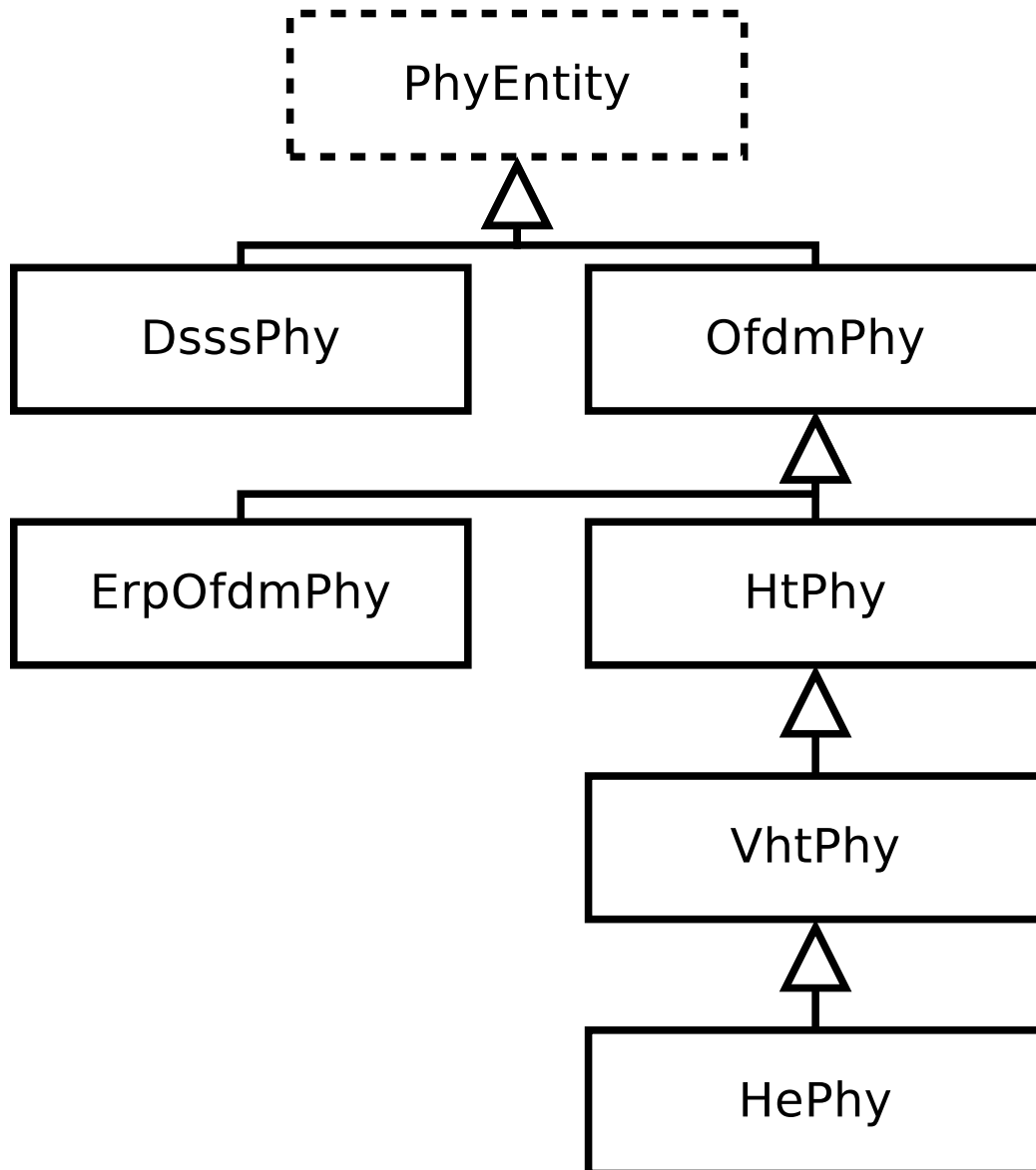
Fig. 2: PhyEntity hierarchy
