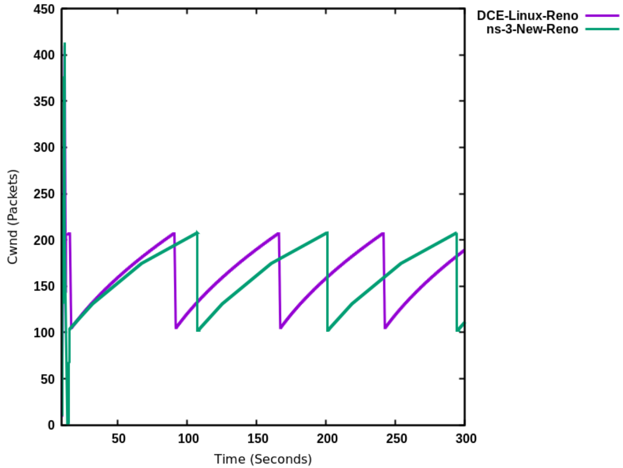
Fig. 8: DCE Linux Reno v/s ns-3 Linux Reno
